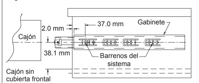
Figura 2 Sistema de 32 mm—Gabinete
