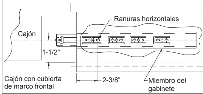
Figura 2 Sistema de 32 mm—Gabinete
